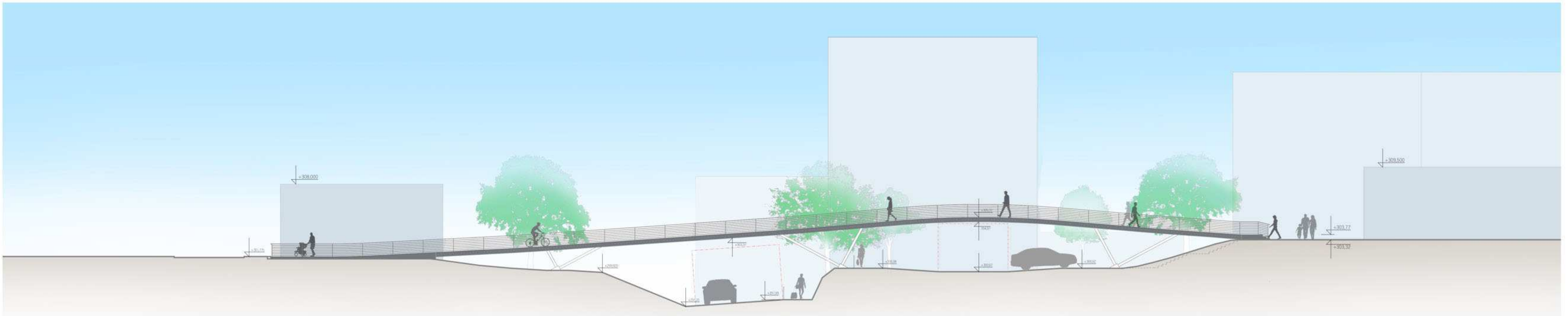
ŘEZ PODÉLNÝ 1:200
