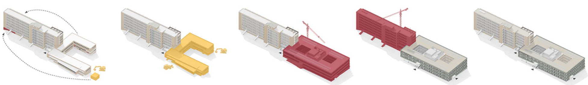
1. Přesun trafostanice a výměníkové stanice do 2PP výškové části 2. Demolice přízemní části polikliniky za provozu výškové části 3. Realizace přístavby za provozu výškové části 4. Rekonstrukce výškové části za provozu přístavby 5. Finální provoz celku
