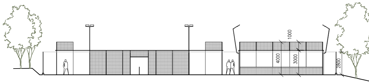
ŘEZ PŘÍČNÝ – SEVER/JIH
