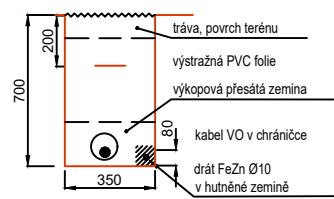
Typový řez A-A uložení kabelové trasy ve volném terénu
