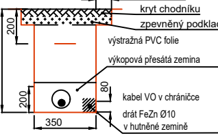
Typový řez B-B uložení kabelové trasy v chodníku
