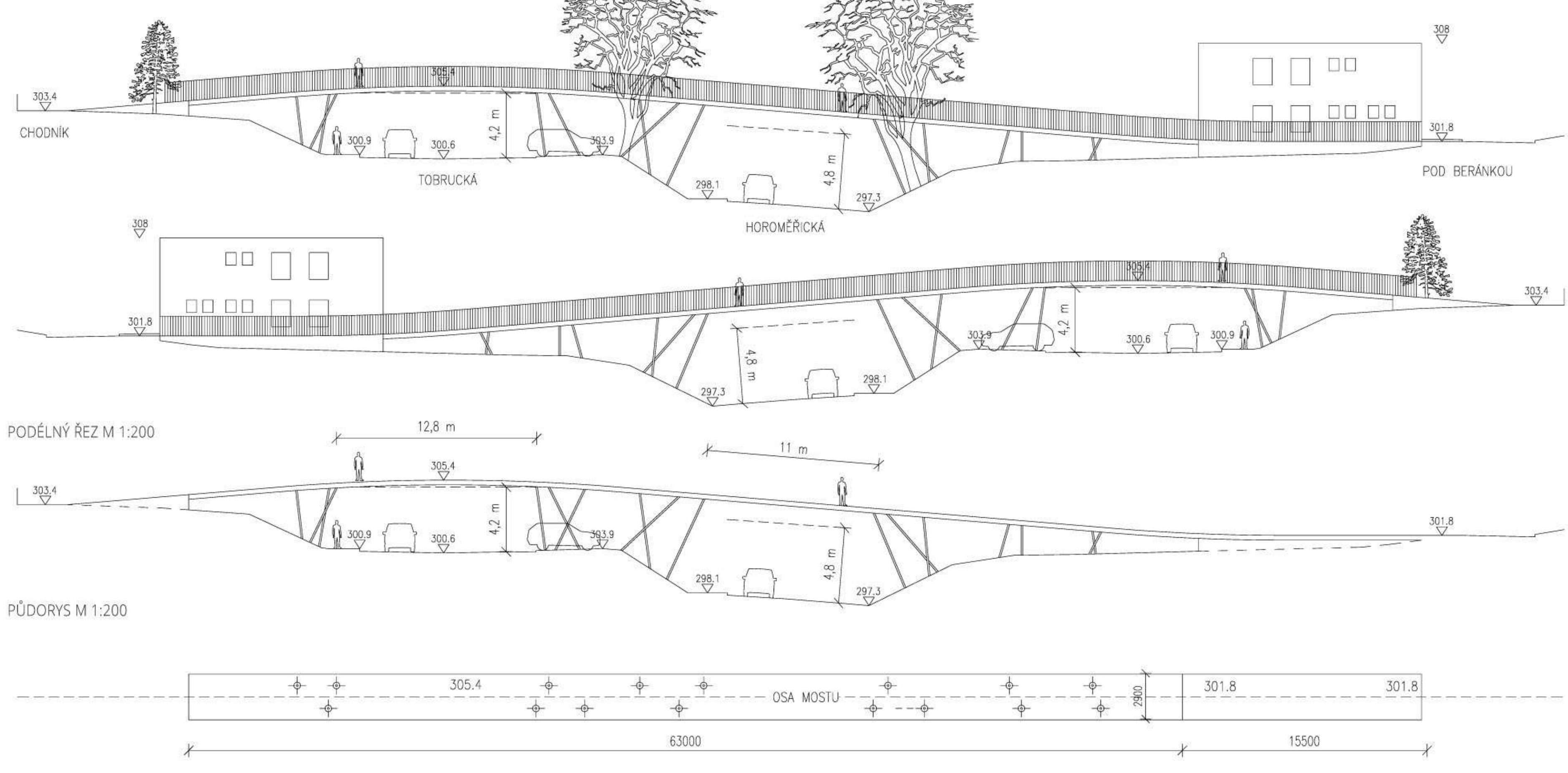
POHLEDY M 1:200
